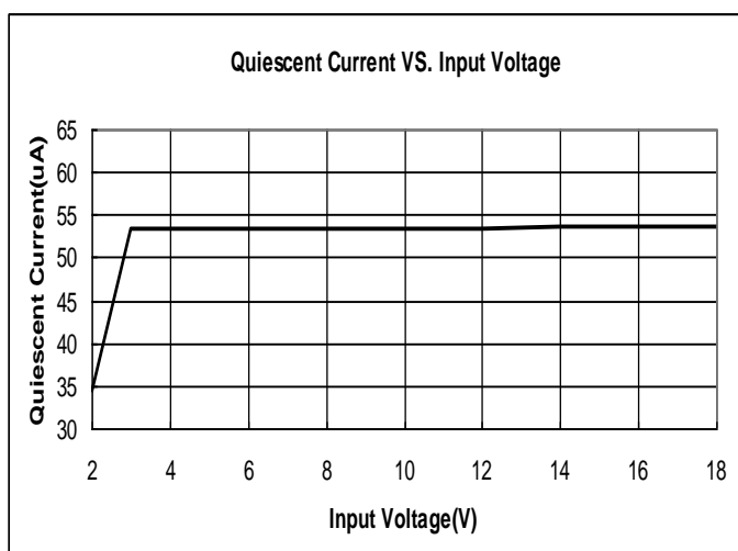
ME6118A25B3G
