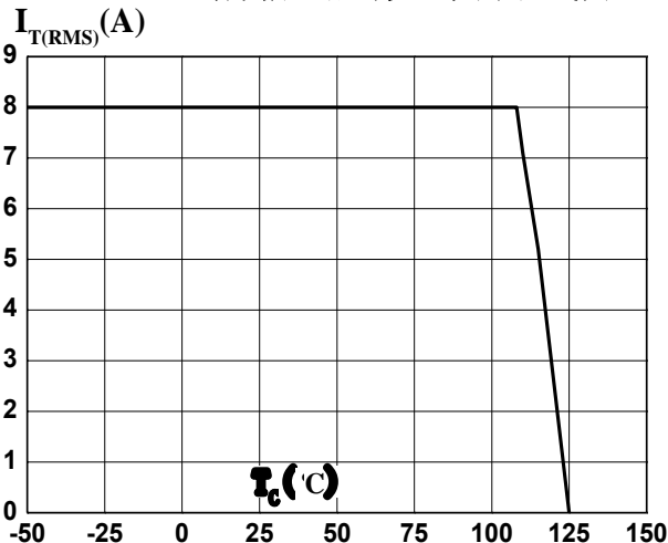
FIG.4: 输出特性图 (最大值图)
