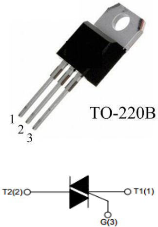
T1:主端子 T2:主端子 G:触发极
